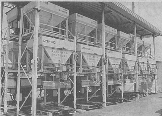
凍結防止剤散布装置。除雪機械と共に雪の多い滋賀に欠かせないアイテム。県内随一の品ぞろえ。必要なときに必要なものだけを貸し出す「レンタルボーイ」も好評
